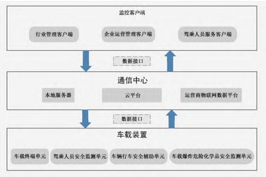
图 1 系统组成示意图
